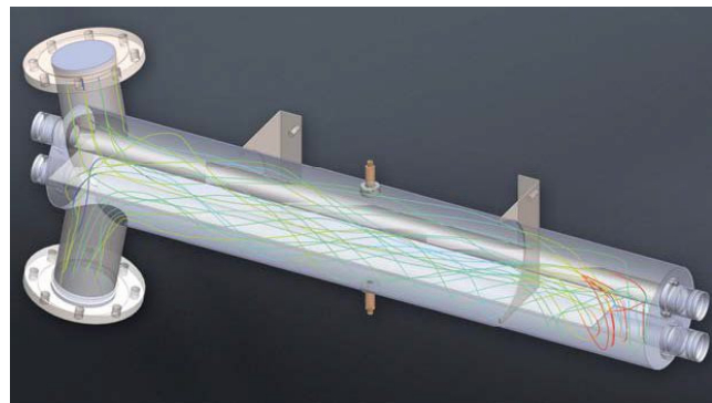
UV ランプ内 流体シミュレーション
