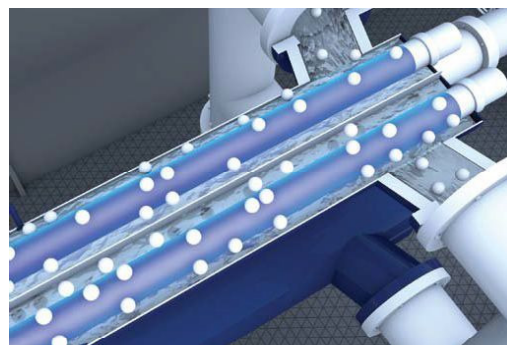
クリーニングボールによる UV ランプの洗浄
